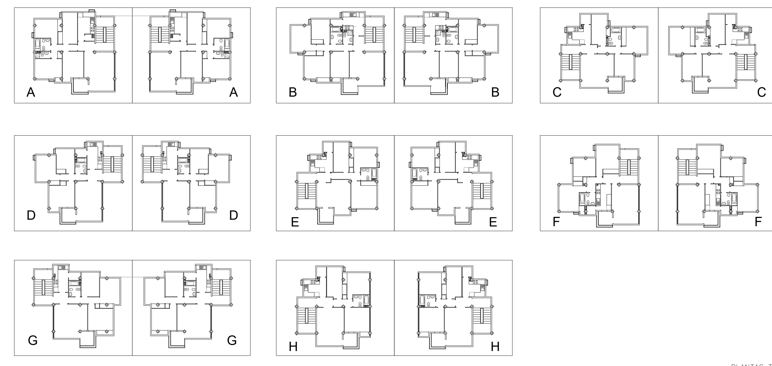
PLANTAS TIPO ESCALA 1:300
